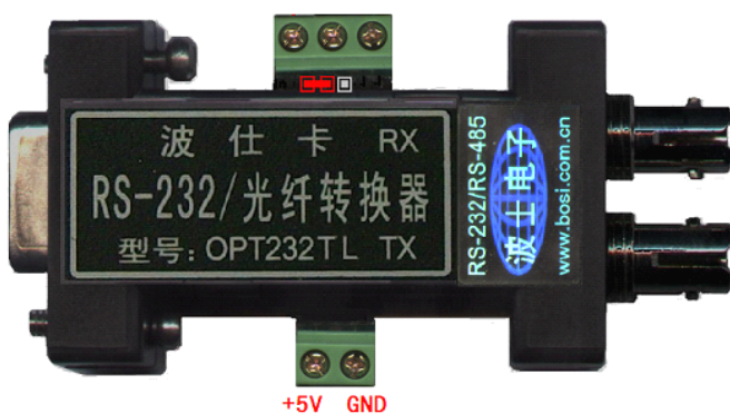
接 RS-232 时
